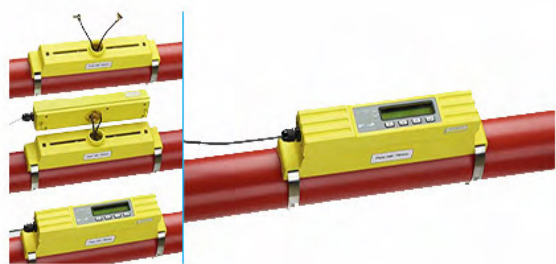
Medidor de Vazão Ultrassônico Compacto Série U1000 FM
